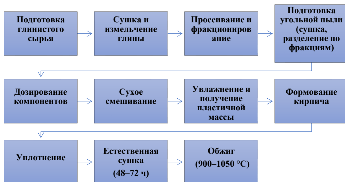
Рисунок 5- Технологическая схема получения керамического кирпича с добавлением угольной пыли
