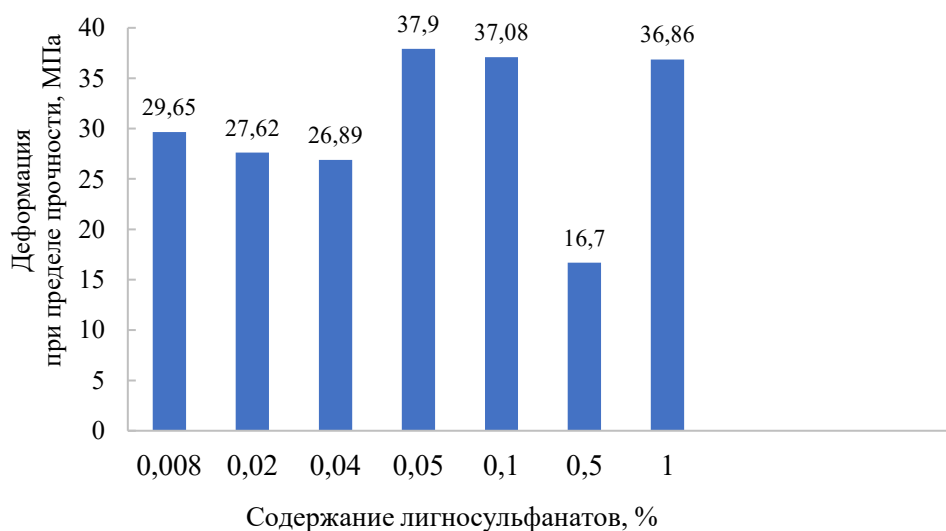
Рисунок 3 – Влияние на деформацию при пределе прочности содержание ЛС в ротационном композите
