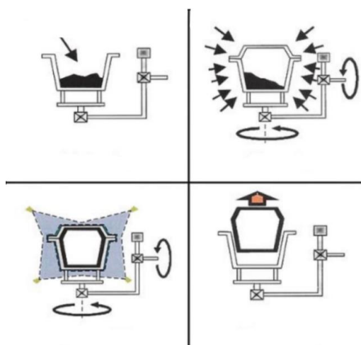
Рисунок 1 - Процесс ротационного формования полимеров [2]
