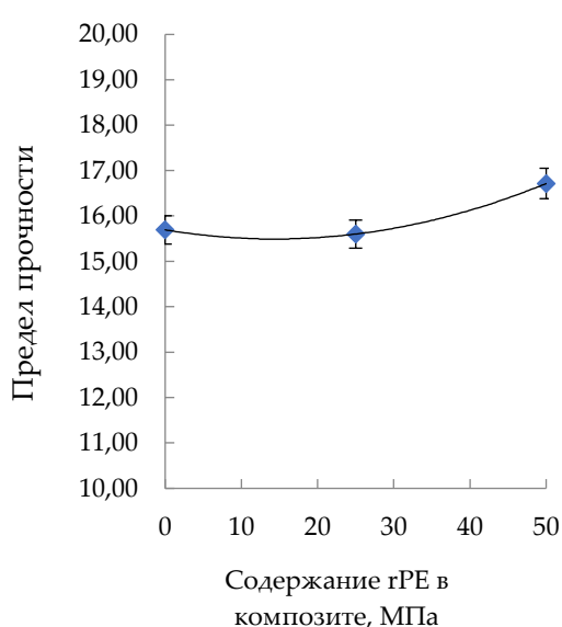
Рисунок 4 – Влияние на пределе прочности содержание вторичного ПЭ и пигмента
