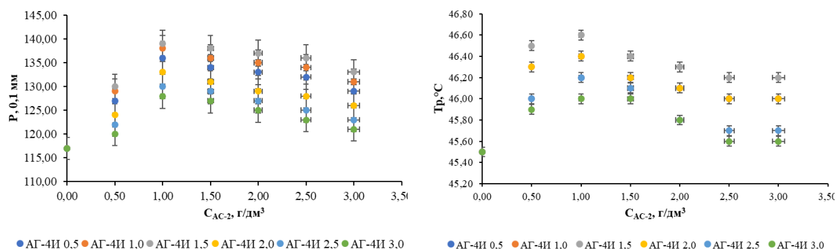
А Б Рисунок 1 – Зависимость глубины проникновения иглы (А) и температуры размягчения (Б) от концентрации модификаторов
