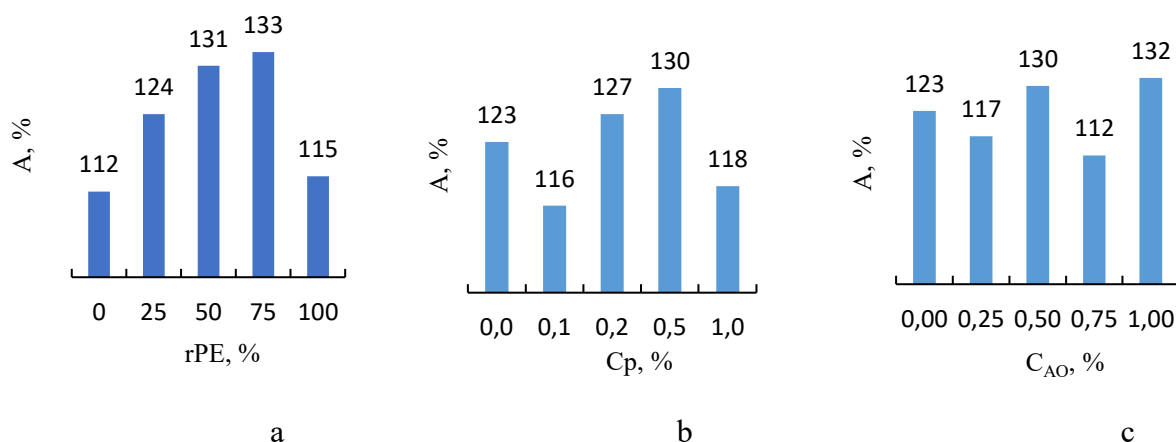
Рисунок 1. Влияние содержания вторичного полиэтилена ( rPE , %) (a), пигмента ( C_p , %) (b) и антиоксидантов ( CAO , %) (c) на амплитуду донного сигнала ( A , %)
