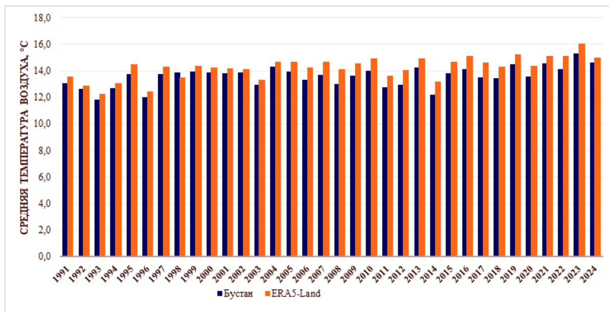
Рисунок 2. Сопоставительная динамика рядов среднемесячной температуры воздуха на метеостанции Бустан и в массиве данных ERA5-Land (1991-2024 гг.)
