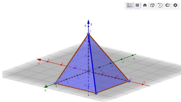
Сурет 3 – GeoGebra бағдарламасындағы есептің визуалды моделі
