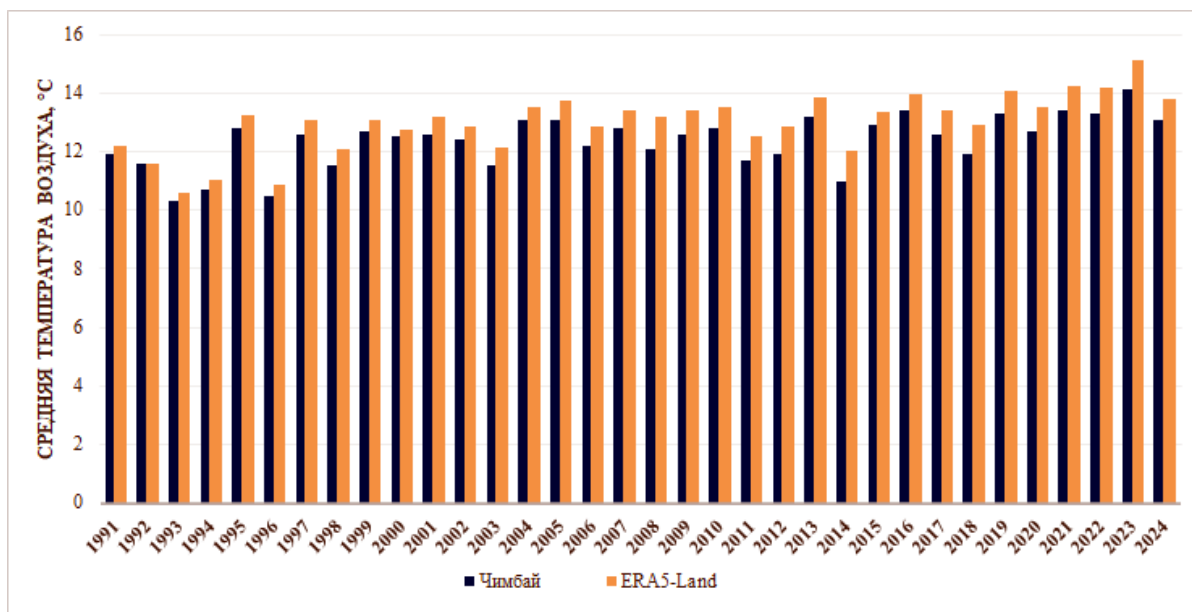
Рисунок 3. Сопоставительная динамика рядов среднемесячной температуры воздуха на метеостанции Чимбай и в массиве данных ERA5-Land (1991-2024 гг.)
