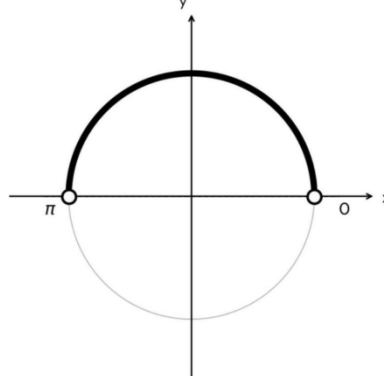
Сурет 23 – \sin x > 0 теңсіздігінің графигі
