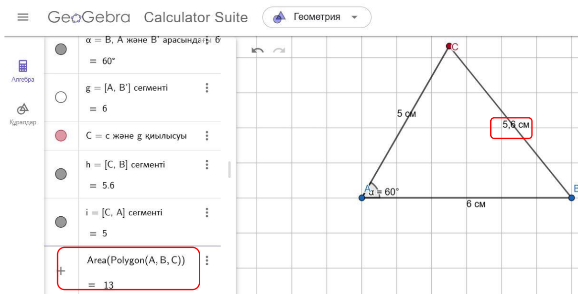
2 сурет атауы: Үшбұрыш ауданы
