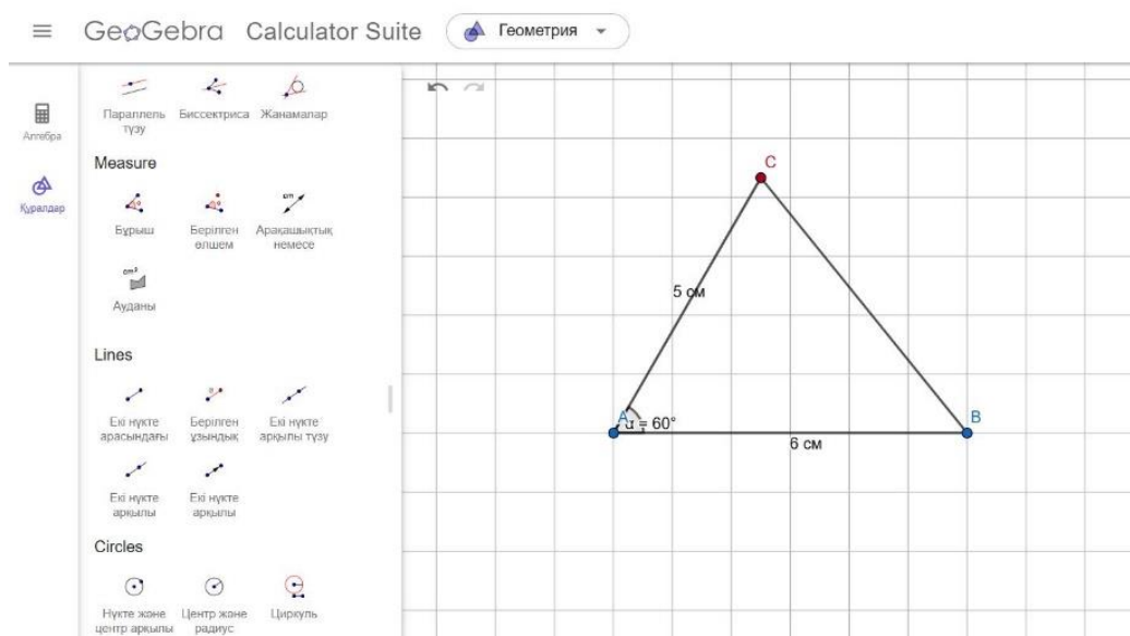
1 сурет атауы: Берілген үшбұрыш
