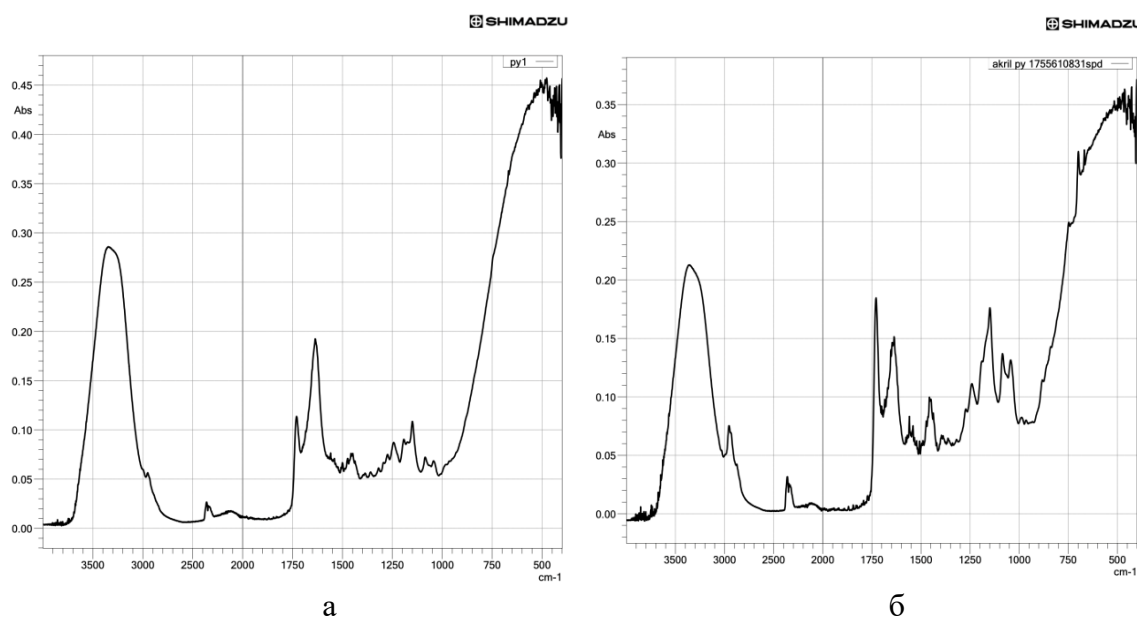
Рисунок 1. ИК-спектры полиуретанового (а) и акрил-полиуретанового (б) пленкообразующих на водной основе
