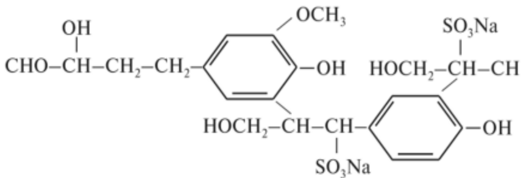
Рисунок 1. Структурная формула промышленного лигносульфаната
