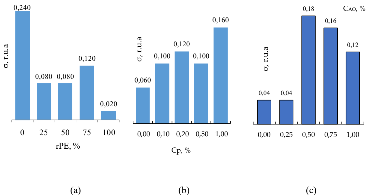
Рисунок 2. Влияние содержания вторичного полиэтилена (гРЕ, %) (а), пигмента (Ср, %) (б) и антиоксидантов (САО, %) (с) на коэффициент пятой гармоники ( \sigma )
