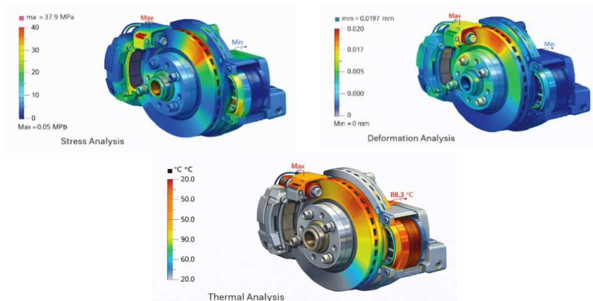
Рисунок 4 – Результаты численного моделирования
