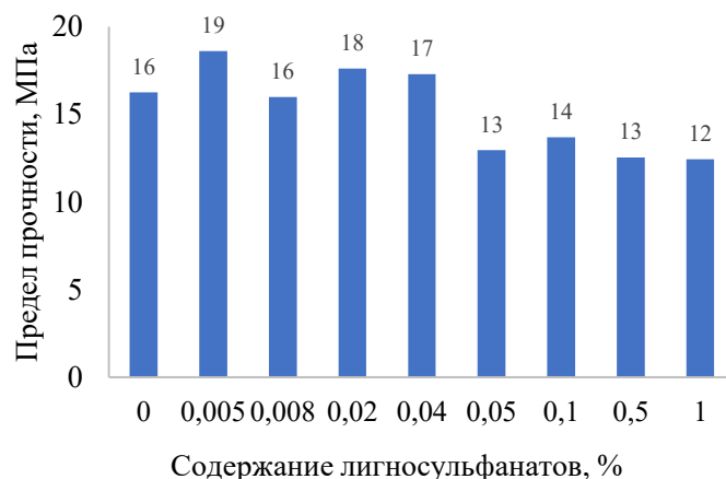
Рисунок 2 – Влияние на предел прочности содержание ЛС в ротационном композите
