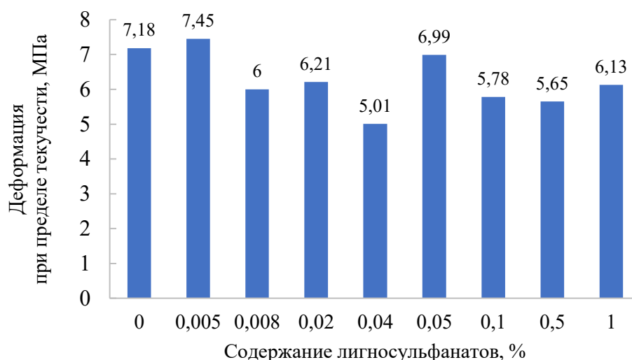
Рисунок 4 – Влияние на деформацию при пределе текучести содержание ЛС в ротационном композите
