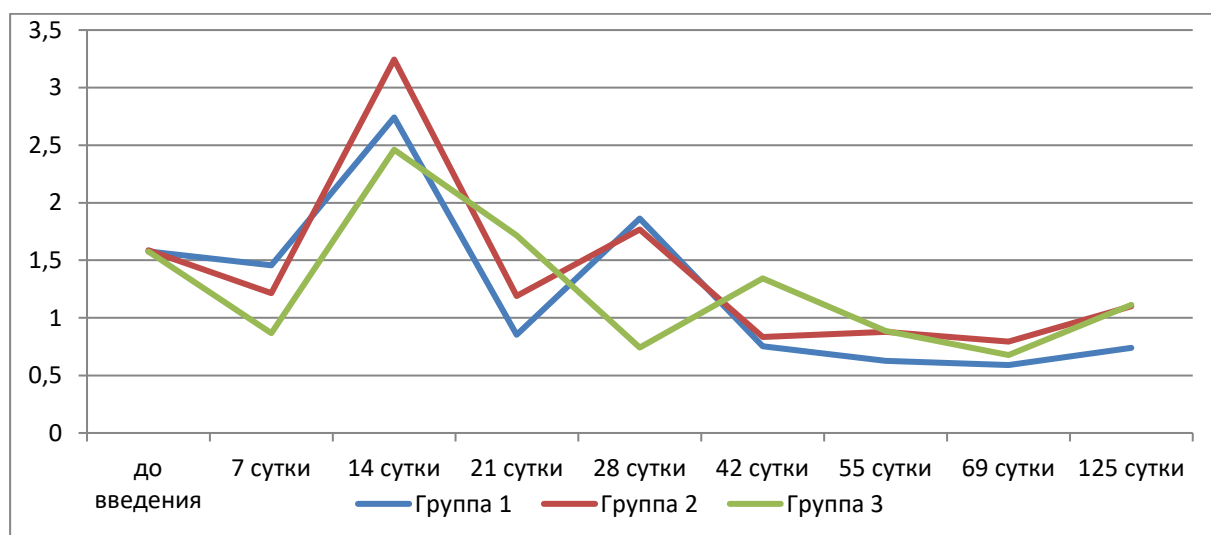
Рисунок 1. - Динамика КС катионных белков нейтрофилов у иммунизированных морских свинок
