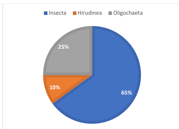
Рисунок 1 – Относительная численность групп организмов зообентоса
