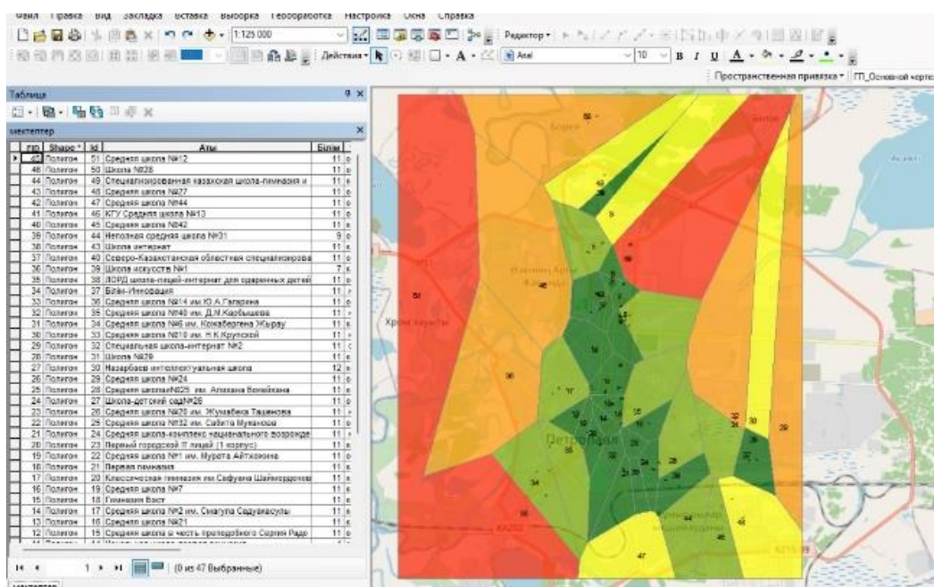
Сурет 3. ArcGIS-та Тиссен көпбұрыштарының құрылысы
