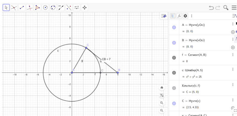
Сурет 1 – GeoGebra бағдарламасындағы есептің сызбасы
