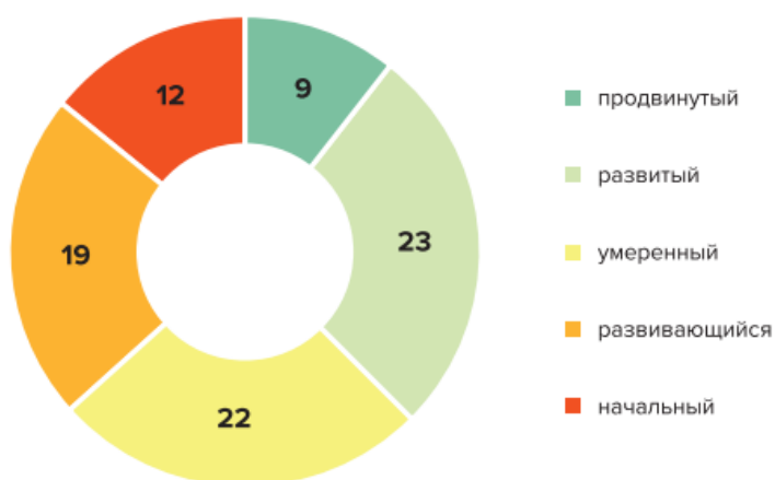
Рисунок 3. Дифференциация 85 регионов РФ по уровню интеграции ESG-критериев в деятельность субъекта [3]
