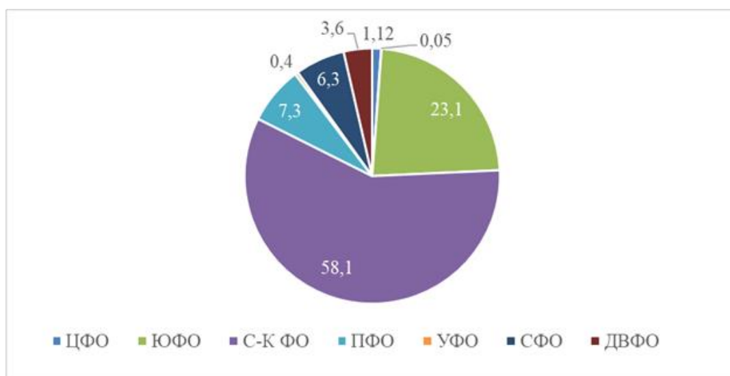
Рисунок 2 – Процент выявленных неблагополучных пунктов по бруцеллезу крупного рогатого скота в федеральных округах от общего количества зарегистрированных в Российской Федерации за 2015-2024 гг
