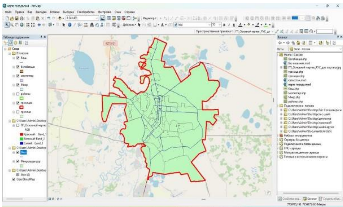
Сурет 1. Петропавл қала шекараларының қабатын құру
