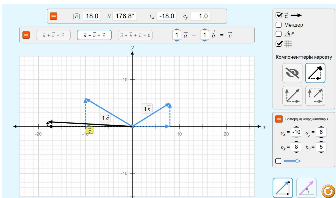
4 сурет атауы: Екі вектордың айырымының мәні
