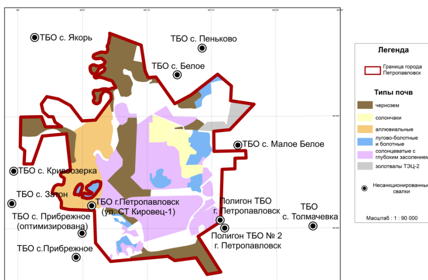
Рисунок 2- Типы почв и размещение полигонов ТБО в окрестностях г.Петропавловска
