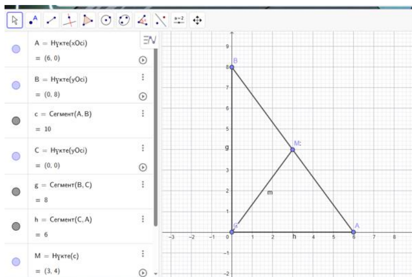
Сурет 2 – GeoGebra бағдарламасындағы есептің визуалды моделі
