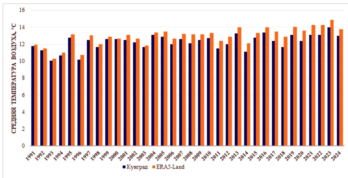
Рисунок 1. Сопоставительная динамика рядов среднемесячной температуры воздуха на метеостанции Кунград и в массиве данных ERA5-Land (1991-2024 гг.)
